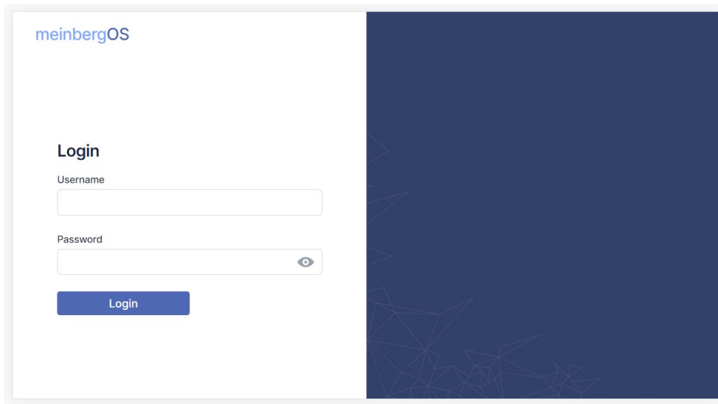
Abbildung 10.1: meinbergOS-Webinterface – Login-Seite
